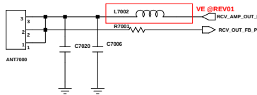
RCV CONTACT
