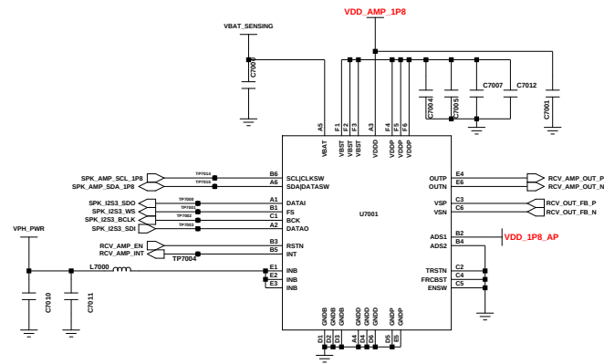
RCV AMP
